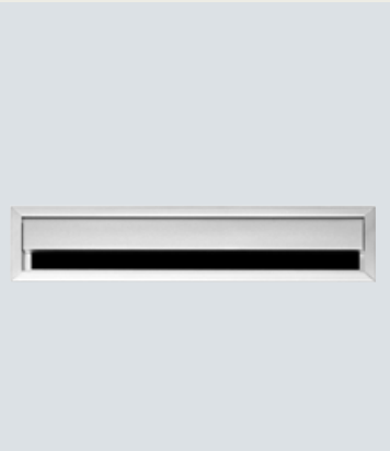
| D | Kabeldurchlass Alu 300 x 70 mm mit Klappe und Bürstendichtung, Durchlass: 270 x 40 mm | E | Wiring grommet, aluminium, 300 x 70 mm, with lid cover and brush seal, opening 270 x 40 mm | F | Passe-câble alu 300 x 70 mm avec clapet et joint-brosse d'étanchéité, passage : 270 x 40 mm | I | Passacavi in alluminio 300 x 70 mm con sportello e guarnizione a spazzola, passaggio: 270 x 40 mm
